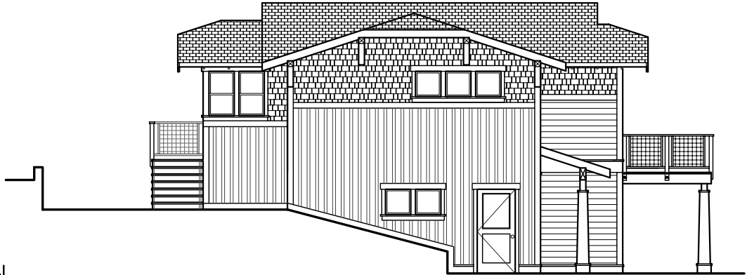
RIGHT ELEVATION
