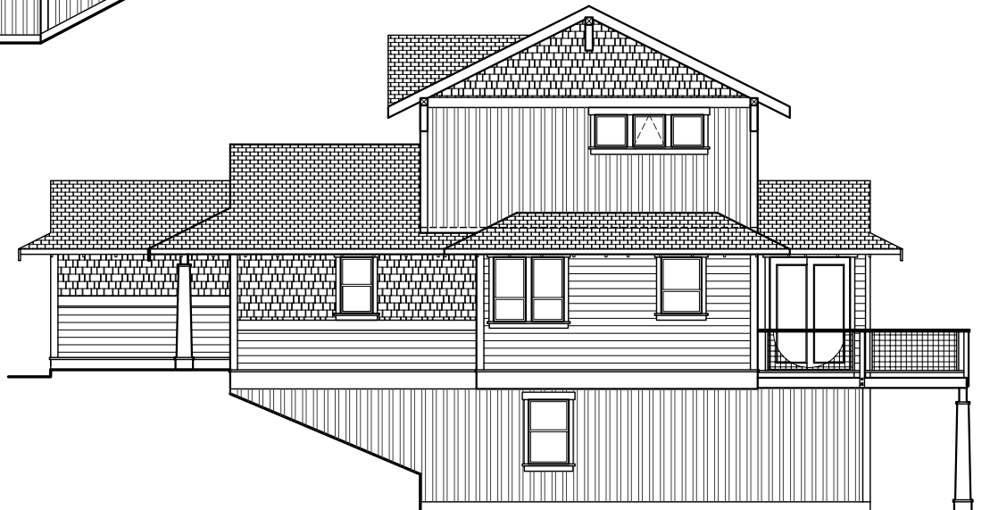
RIGHT ELEVATION
